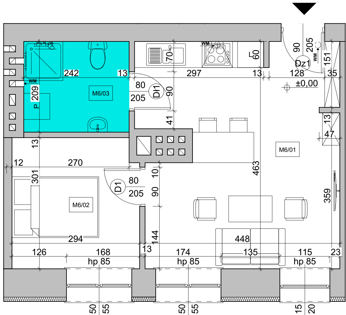
RZUT MIESZKANIA 1:50
