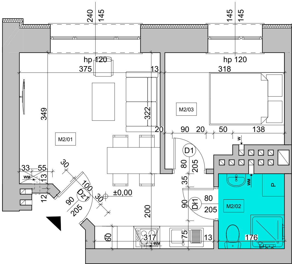
RZUT MIESZKANIA 1:50
