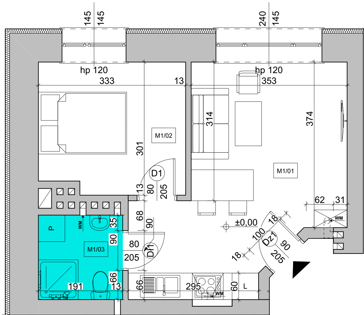
RZUT MIESZKANIA
